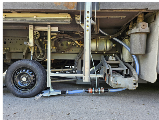
Verbaute Messkonstruktion im MoReLab
